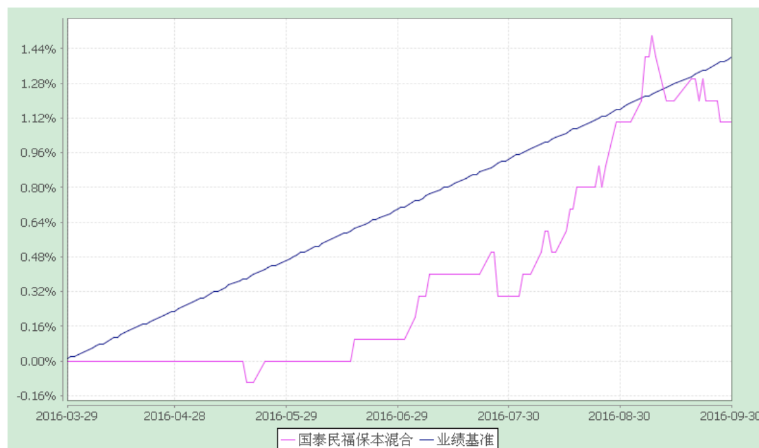
国泰民福保本混合型证券投资基金 累计净值增长率与业绩比较基准收益率历史走势对比图 (2016 年 3 月 29 日至 2016 年 9 月 30 日)
